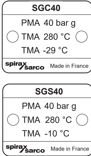
Fig. 2 Standard name-plates
